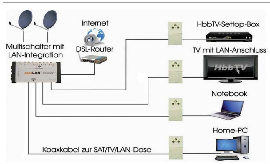
Abbildung 1: Ein Netz - zwei Funktionen: HF und IP über eine gemeinsame koaxiale sternförmige Verteilstruktur.
