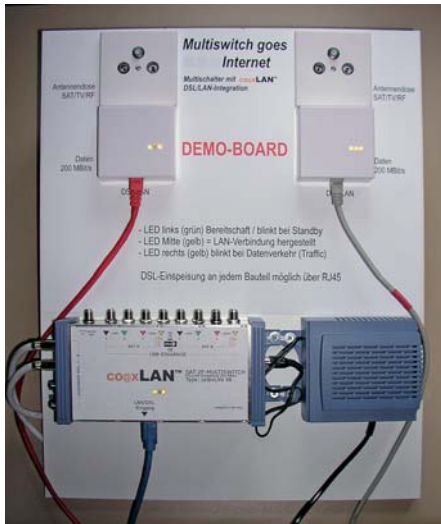
Abbildung 2: Mit den Komponenten einer Vorserien-Demotafel lässt sich das Potential der co@xLAN-Technik hervorragend erkennen.
